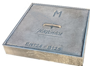
Tapa tipo M homologada Telefónica
