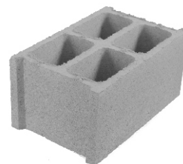
bloque normal 25 x 40 (2 camaras)
