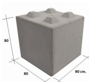
Blokazo 80 media pieza
