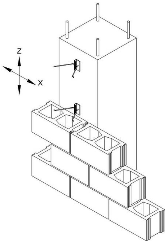
ANCLAJE CON TIRO AL PILAR DE HORMIGÓN ARMADO CON 2 LIBERTADES DE MOVIMIENTO
