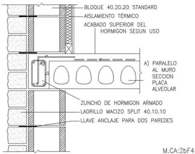
■ Fig.IV.2.2g. Secciones de encuentro de muro doble de ladrillo y BHH con forjado de placas alveolares cargando en hoja interior: S. transversal a la placa; S. longitudinal a la placa. M.CA: 2bF4
