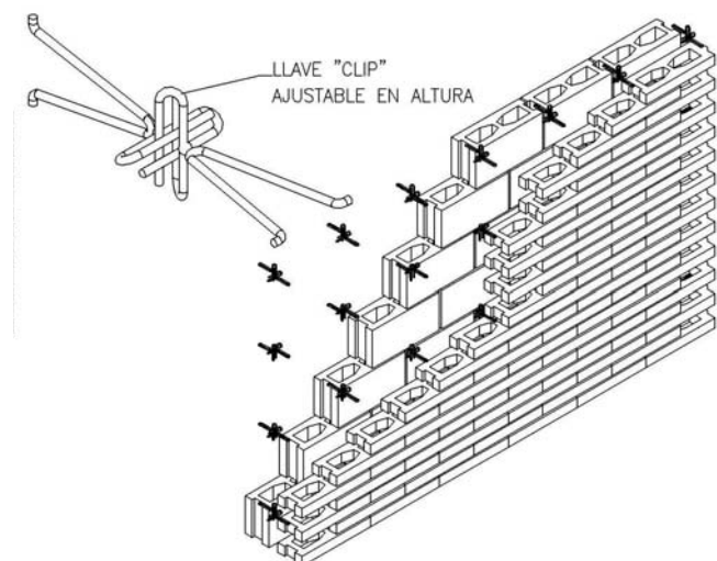
■ Fig.II.2.4 Muro de dos hojas de piezas distintas, con llaves ajustables en altura.
