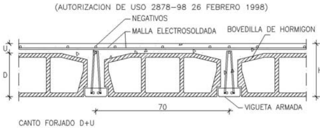
FIG.III.2.1.1a. SECCIÓN TRANSVERSAL CON VIGUETAS Y BOVEDILLAS
