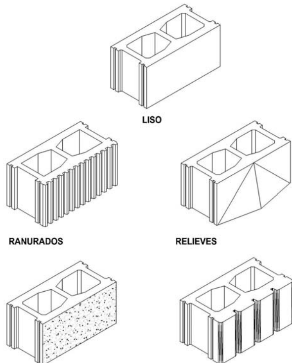
■ Fig.I.1.1e. Acabados del bloque de hormigón visto.
