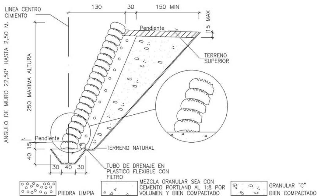
FIG.III.4a. ESQUEMA DE MURO DE CONTENCIÓN CON SILLARES DE HORMIGÓN ATIRANTADOS
