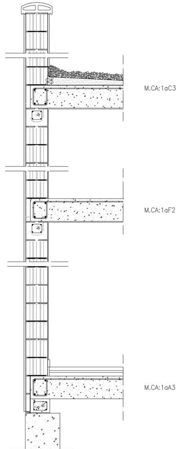
■ Fig.IV.2.1b. Sección de encuentro de muro de 1 hoja de bloque de árido ligero de carga (Arliblock). M.CA: 1aA3 / M.CA: 1aF2 / M.CA: 1aC3
