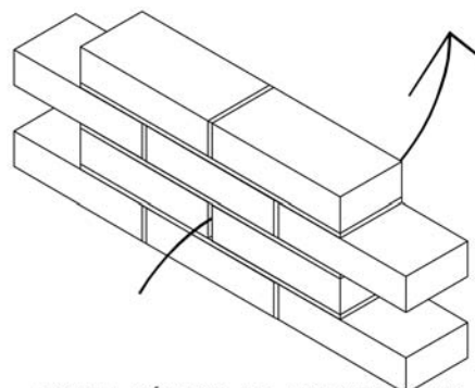
■ Fig. I.5.d Cámaras de aire ventiladas.
