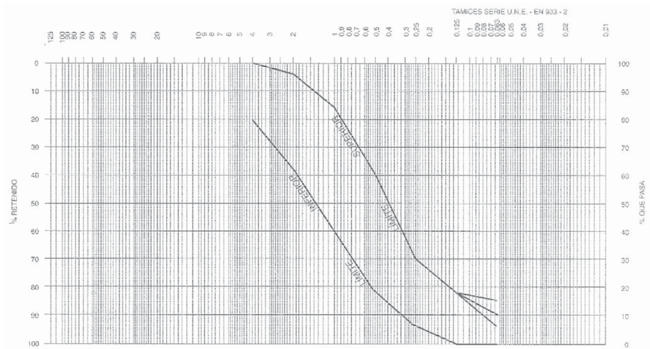
■ Fig.1.2.1c. Huso granulométrico del árido fino
