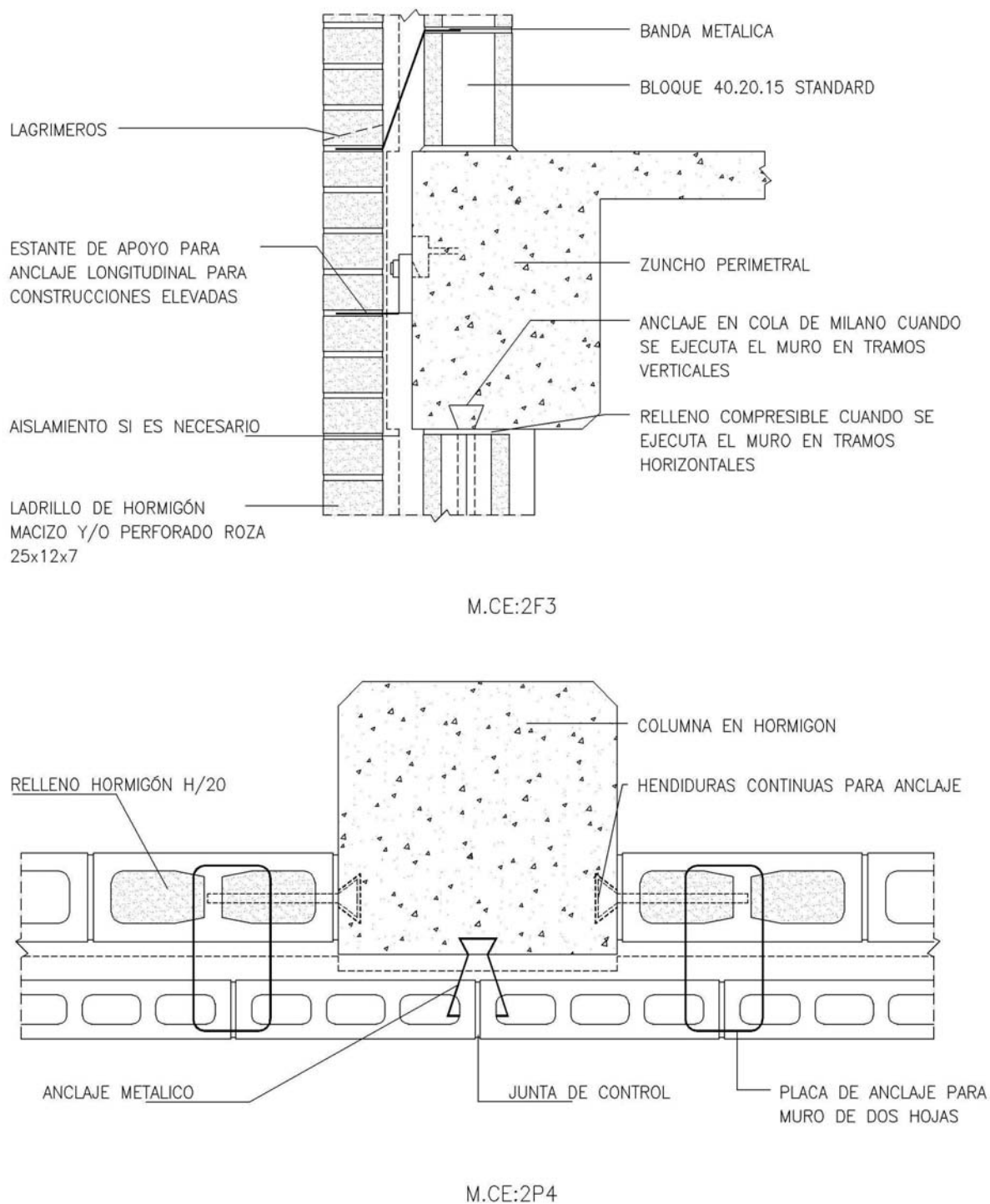
■ Fig.IV.1.2d. Planta y sección de encuentros de muro de 2 hojas de ladrillo y BHH de cerramiento. Hoja exterior de ladrillo de hormigón pasante y apoyada en angular. Hoja interior de bloque de hormigón hueco fijada a soportes. M.CE: 2F3 / M.CE: 2P4
