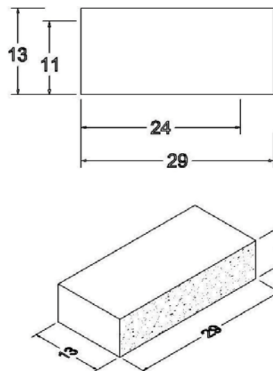
■ Fig.I.1.3a. Ladrillo macizo de Hormigón normal
