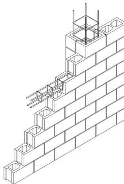
■ Fig.II.3.2a Muro con piezas especiales para pilastra sobresaliente de hormigón armado.
