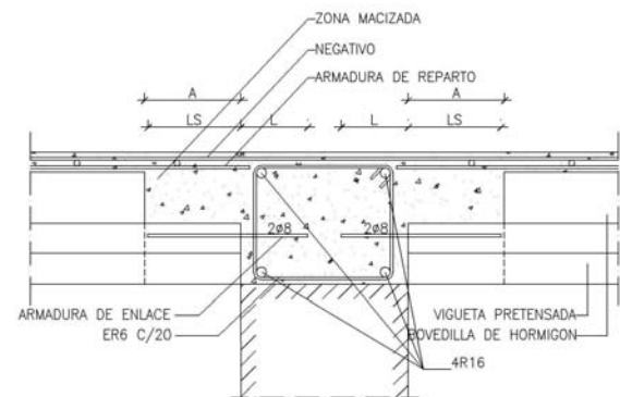
FIG.III.2.1.2a. SECCIÓN TRANSVERSAL CON SEMIVIGUETAS PRETENSADAS Y BOVEDILLAS
