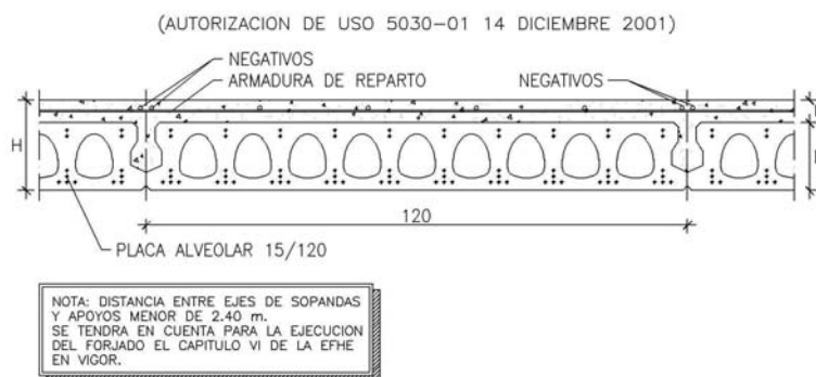
FIG.III.2.1.3.1a. SECCIÓN TRANSVERSAL CON PLACAS ALVEOLARES
