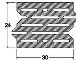
■ Fig.I.1.1d. Bloque multicámara machihembrado de árido denso y sin machihembrar
