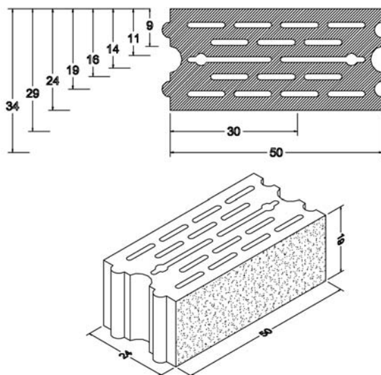
■ Fig.I.1.2a. Bloque Arliblock Macizo
