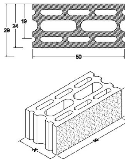
■ Fig.I.1.2b. Bloque Arliblock MultiCámara
