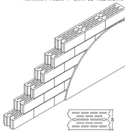
FIG.V.3f. MURO DE 1 HOJA DE BLOQUE DE HORMIGÓN ALIGERADO (ARLIBLOCK)
