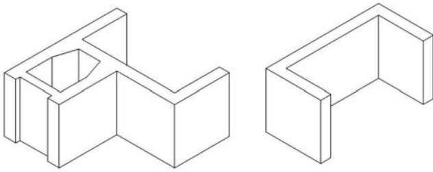
■ Fig.I.1.1b4. Bloques pilastra de enlace y pilastra sencilla.
