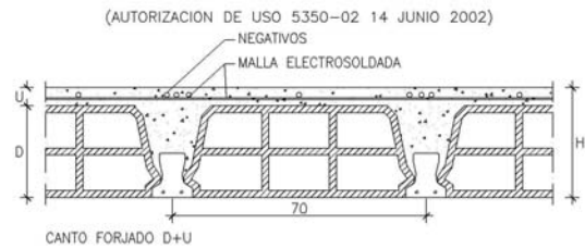
FIG.III.2.1.2a. SECCIÓN TRANSVERSAL CON SEMIVIGUETAS PRETENSADAS Y BOVEDILLAS
