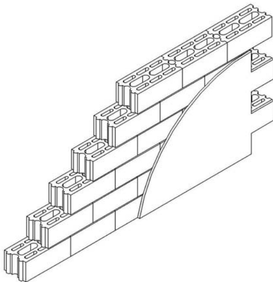
■ Fig.II.2.2 Muro enfoscado de árido ligero multicámara.
