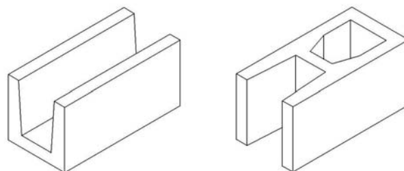
■ Fig.I.1.1b2. Bloques en "U" para crear zunchos o vigas de hormigón armado.
