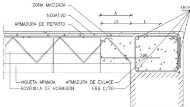
FIG.III.5.1b. SECCIÓN POR EL APOYO SOBRE MURO INTERMEDIO
