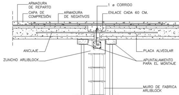
FIG.III.2.1.3.2b. SECCIÓN POR LA JUNTA ENTRE PLACAS ALVEOLARES SOBRE MURO INTERMEDIO
