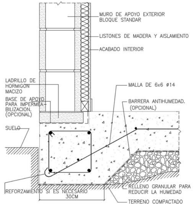
■ Fig.IV.2.1d. Secciones de arranque de muro de 1 hoja de BHH de carga sobre cimentación de losa flotante. M.CA: 1bA1
