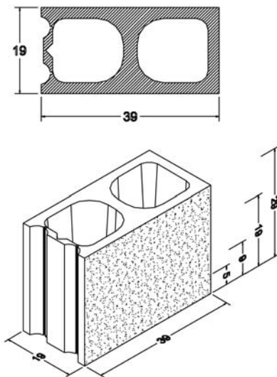
■ Fig.I.1.1c. Bloque Universal
