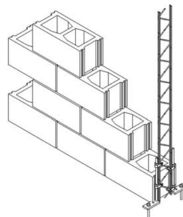
2 FIJACIONES AL PIE EN MURO EN MÉNSULA
