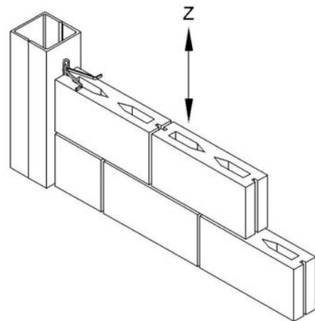
MURO ENTESTADO A PILAR METÁLICO Y ANCLADO CON UNA LIBERTAD DE MOVIMIENTO
