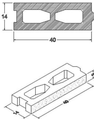
■ Fig.I.1.3b. Ladrillo hueco de Hormigón alargado
