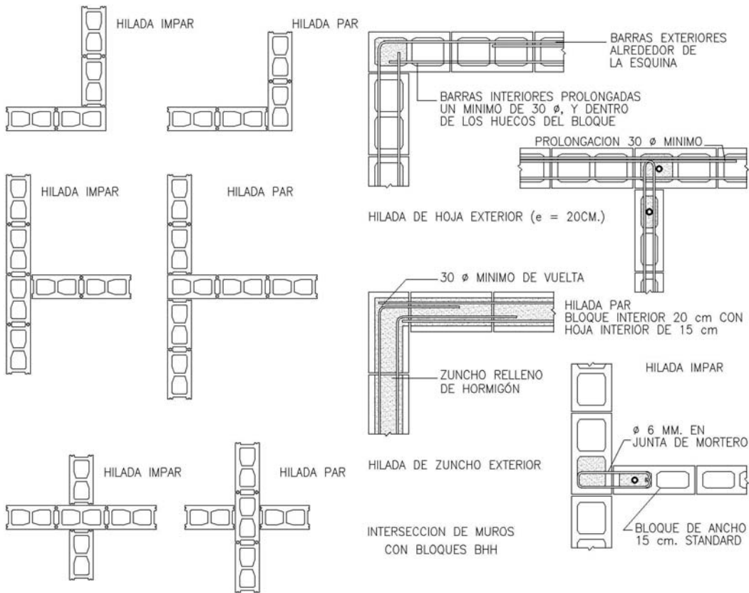
FIG.II.6.1a. ENCUNTROS DE MUROS SIN ARMAR
