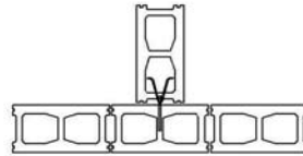
FIG.III.4.3b. ENCUESTRO DE MURO DE CARGA CON MURO DE ARRIOSTRAMIENTO CON ANCLAJE QUE SÓLO PERMITE EL LIBRE MOVIMIENTO VERTICAL
