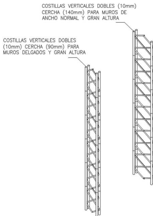
■ Fig.1.3.3.c Costillas verticales de refuerzo prefabricadas: tipo cercha sencilla duplicada.
