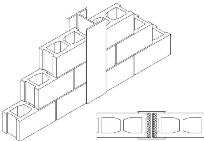
■ Fig.IV.2.3a. Muros de bloque de hormigón confinados entre pilares y vigas de hormigón armado.
