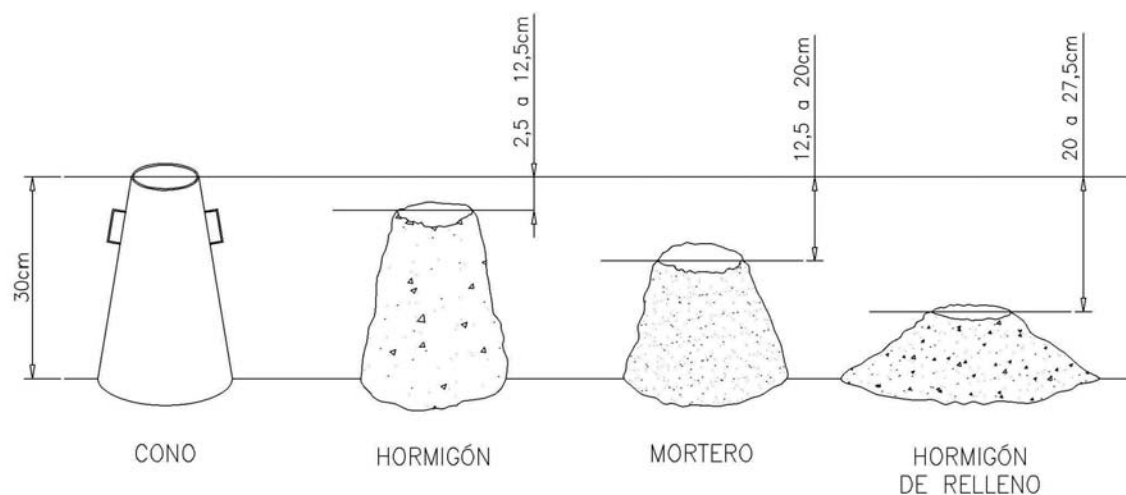
■ Fig.I.2. Diferencias de plasticidad entre hormigón en masa, mortero y hormigón de relleno.
