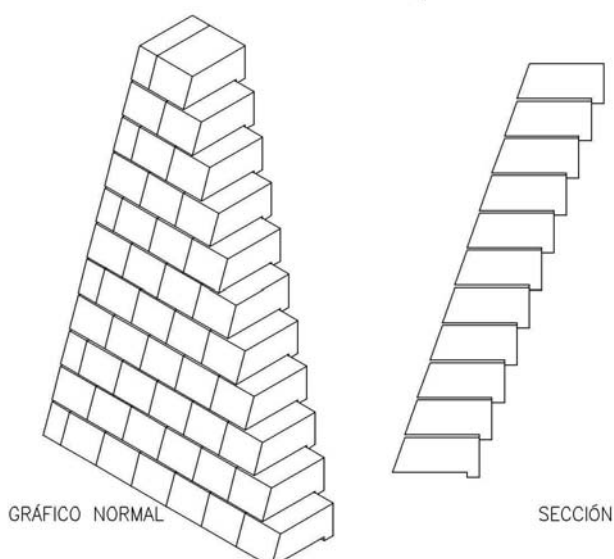
■ Fig.II.2.5 Muro de sillares prismáticos de hormigón.
