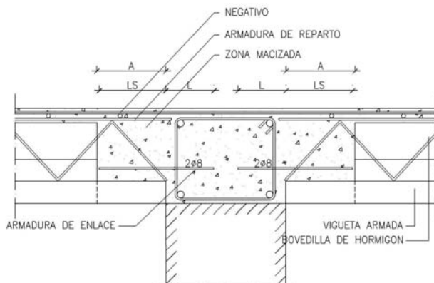
FIG.III.2.1.1a. SECCIÓN TRANSVERSAL CON VIGUETAS Y BOVEDILLAS
