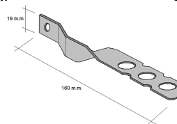
anclaje muro pasante
