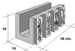
dintel
