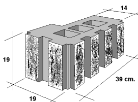
esquina
