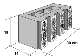
caras lisas
