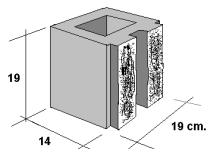
medio
